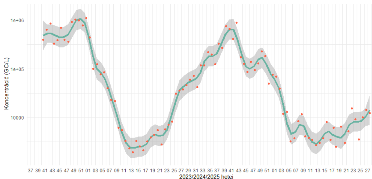
1. ábra A szennyvízben mért SARS-CoV-2 kópiaszám országos, lakosságáramnyos súlyozott átlaga. A véletlenszerű ingadozások hatásának kiszűrése érdekében nem-parametrikus regressziós LOWESS (LOcally WEighted Scatter-plot Smoother) módszer felhasználásával létrehozott simított görbe (zöld). A piros pontok a nyers adatokat mutatják, a szürke sáv a 95%-os konfidencia-intervallumot jelöli.
